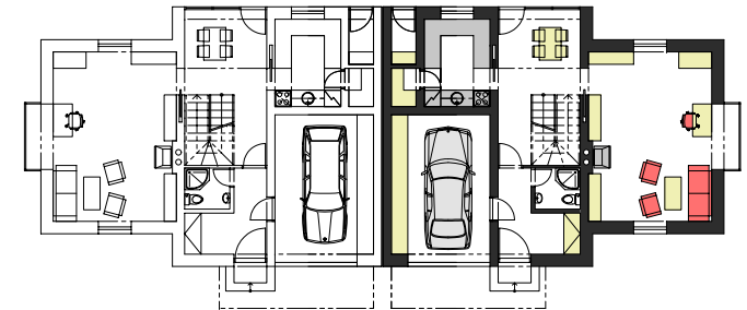
Schéma 1.np - přízemí dvojdomu
